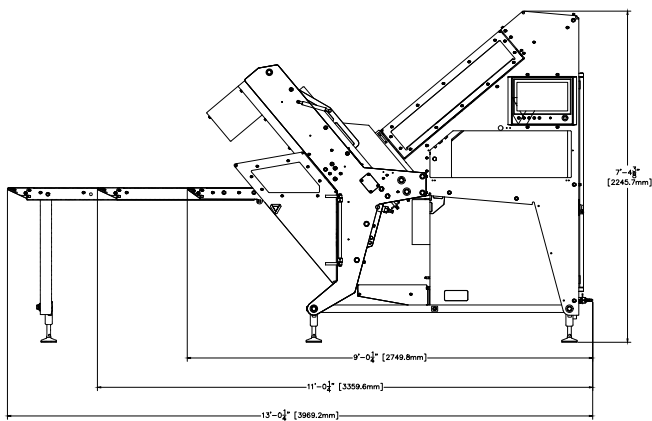
Abtransportband-Optionen
